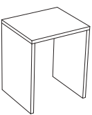
75x65x h91 cm struttura a giorno per inserimento modulo open structure for 1 module
