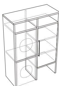
145,6x65x h210 cm colonna con ante porta lavatrice+asciugatrice + ripiani column for washing machine + dryer + shelves
