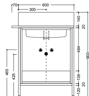
60 BACINO DOPPIA PROFONDITÀ + CONTENITORE ANTE 60 DUAL LEVEL WASHBASIN + CONTAINER WITH DOORS
