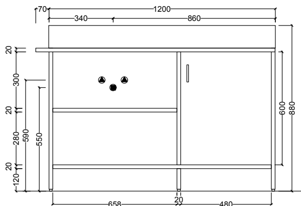
120 BACINO SX + ANTA 120 LEFT WASHBASIN + DOOR
