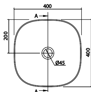
LAVABO DA APPOGGIO QUADRATO 40X40H12,5 CM SQUARE COUNTERTOP WASHBASIN 40X40H12.5 CM
