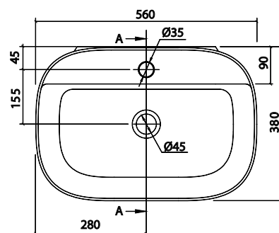
LAVABO DA APPOGGIO OVALE, 56X38H14 CM PREDISPOSTO PER RUBINETTERIA MONOFORO OVAL COUNTERTOP WASHBASIN, 56X38H14 CM LAYOUT FOR SINGLE-HOLE TAPS
