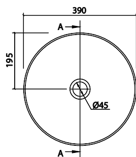
LAVABO DA APPOGGIO TONDO Ø39XH14CM ROUND COUNTERTOP WASHBASIN Ø39XH14CM
