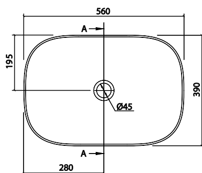
LAVABO DA APPOGGIO OVALE 56X39H14 CM OVAL COUNTERTOP WASHBASIN 56X39H14 CM
