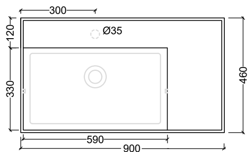
90 BACINO UNICO DOPPIA PROFONDITÀ 90 DUAL LEVEL SINGLE WASHBASIN
