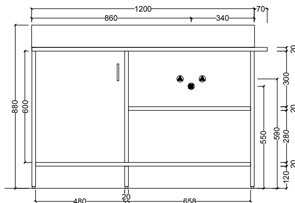
120 BACINO DX + ANTA 120 RIGHT WASHBASIN + DOOR
